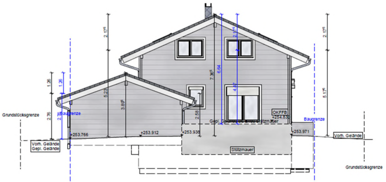
Ansicht West
